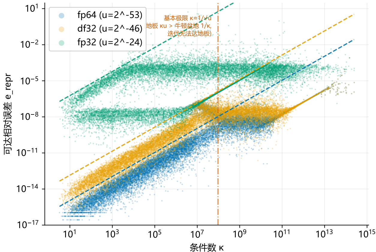
可达精度下限:floorscaled 初值, 三精度各贴 \kappa \cdot u 线(无构造偏置)
