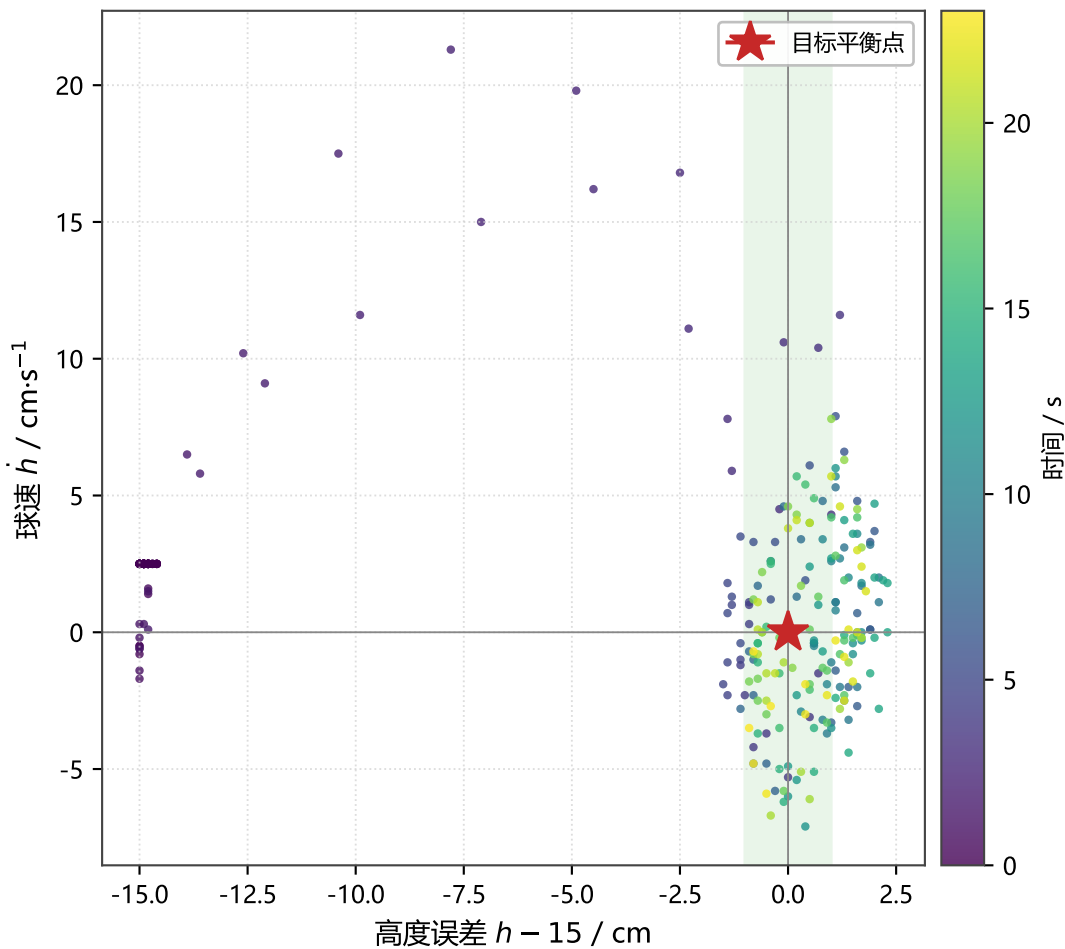
15 cm 定高相轨迹 (收敛到平衡点)
