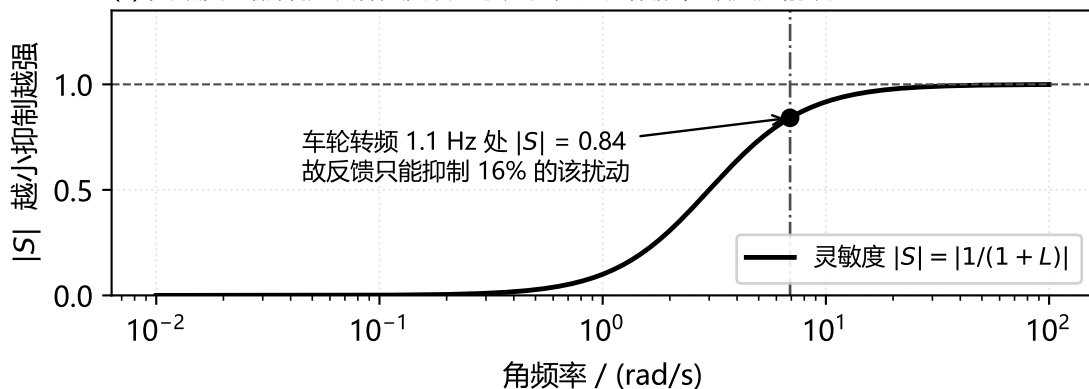
(c) 灵敏度: 俯仰扰动落在反馈几乎无能为力的频段, 故只能前馈
