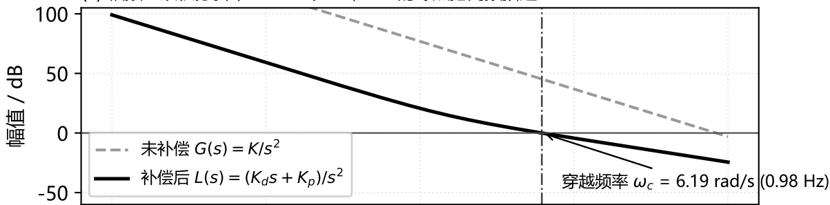
(a) 幅频: 双积分斜率 -40 dB/dec, PD 的零点把高频抬起
