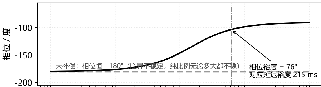
(b) 相频: PD 提供相位超前, 把相角抬高 -180^\circ
