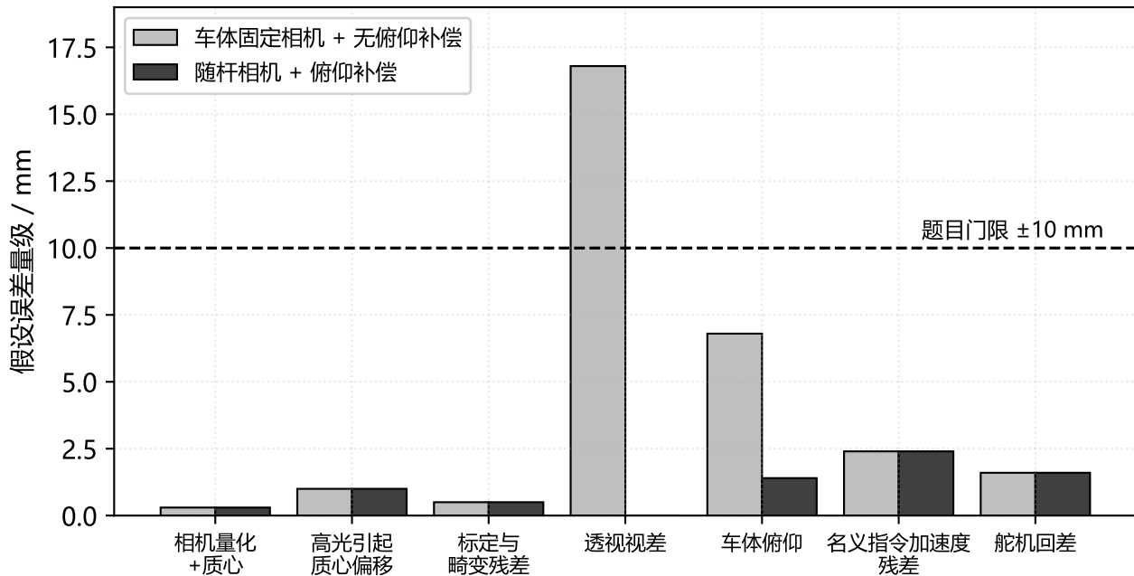
[设计估计] 误差灵敏度 RSS 对比: 18.4 mm 与 3.4 mm (非整机实测)
