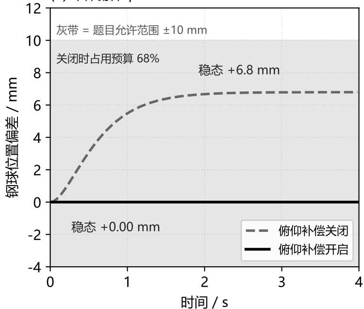
(b) 车体俯仰 \varphi = 0.5^\circ
