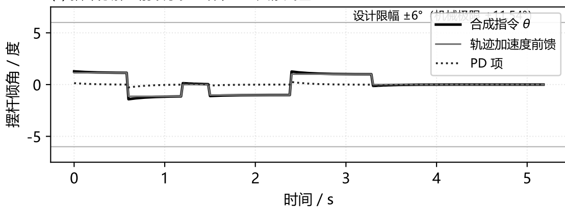
(c) 指令分解: 前馈承担主体, PD 只修残差
