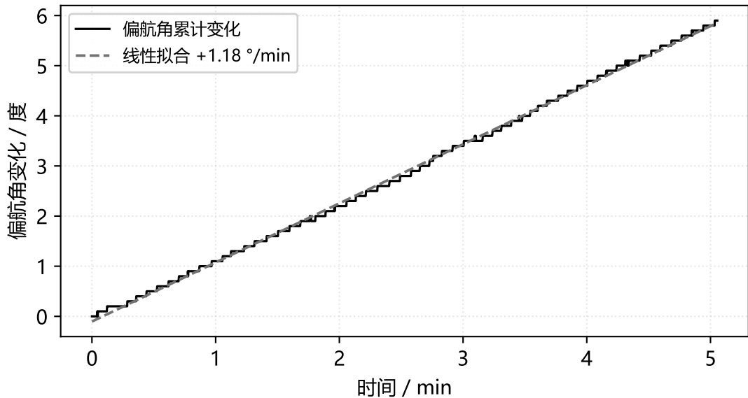
[实测] 静止 5 分钟的偏航积分漂移 (已做零偏标定)
