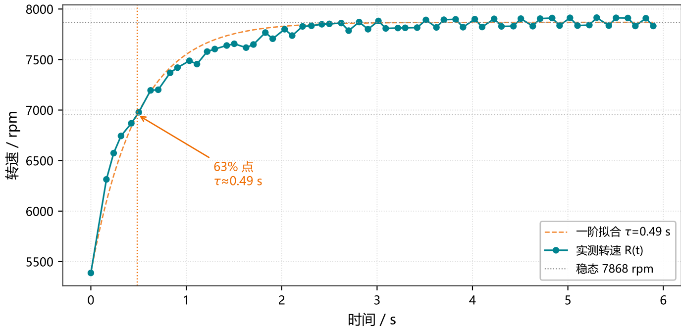
风机阶跃响应与时间常数辨识 (PWM 3000→4000, 暖机段)
