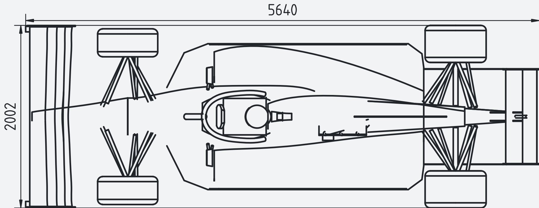
上面図 TOP
