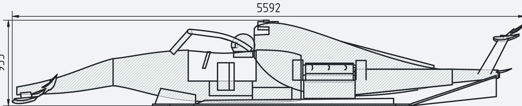
断面 A-A
