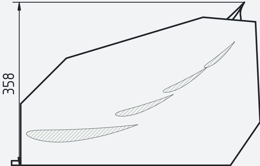
側面図 1:5
