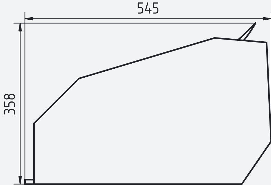
側面図 1:5
