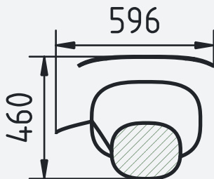
断面 D-D
