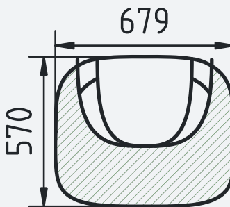
断面 E-E
