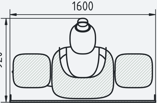
断面 G-G
