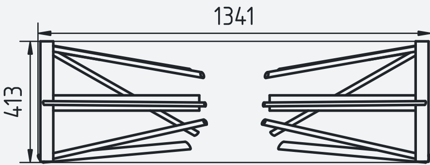
リア 背面図
