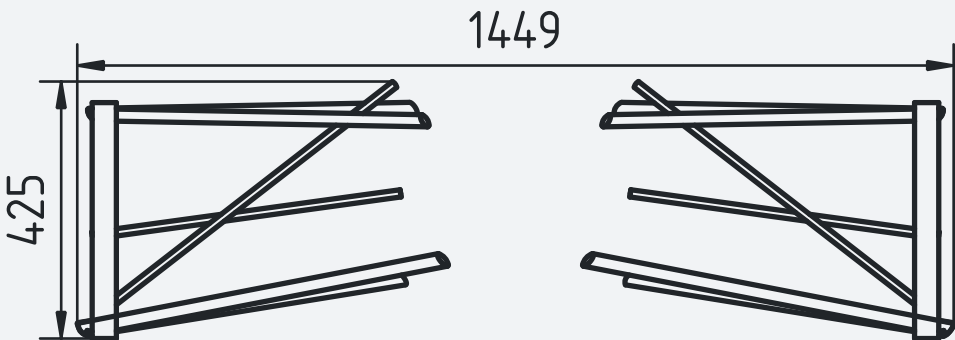
フロント 正面図
