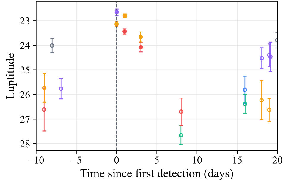
KN | Ndet=6 | Nbands=6 | Nobs=20
