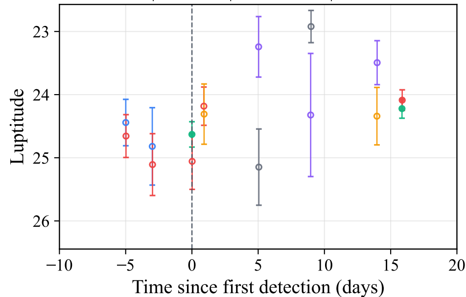
AGN | Ndet=3 | Nbands=6 | Nobs=16
