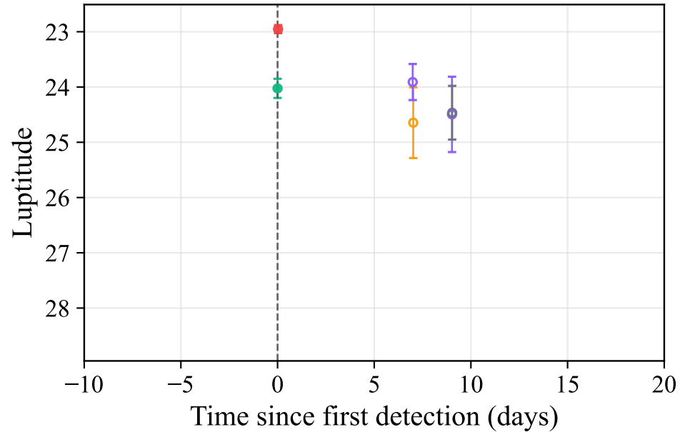
KN | Ndet=2 | Nbands=5 | Nobs=6
