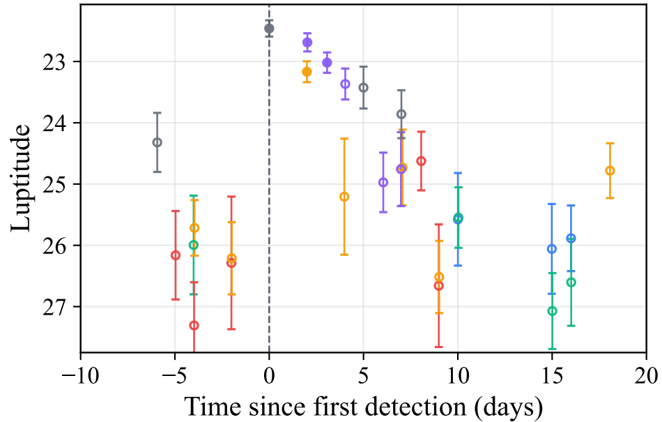
KN | Ndet=4 | Nbands=6 | Nobs=28
