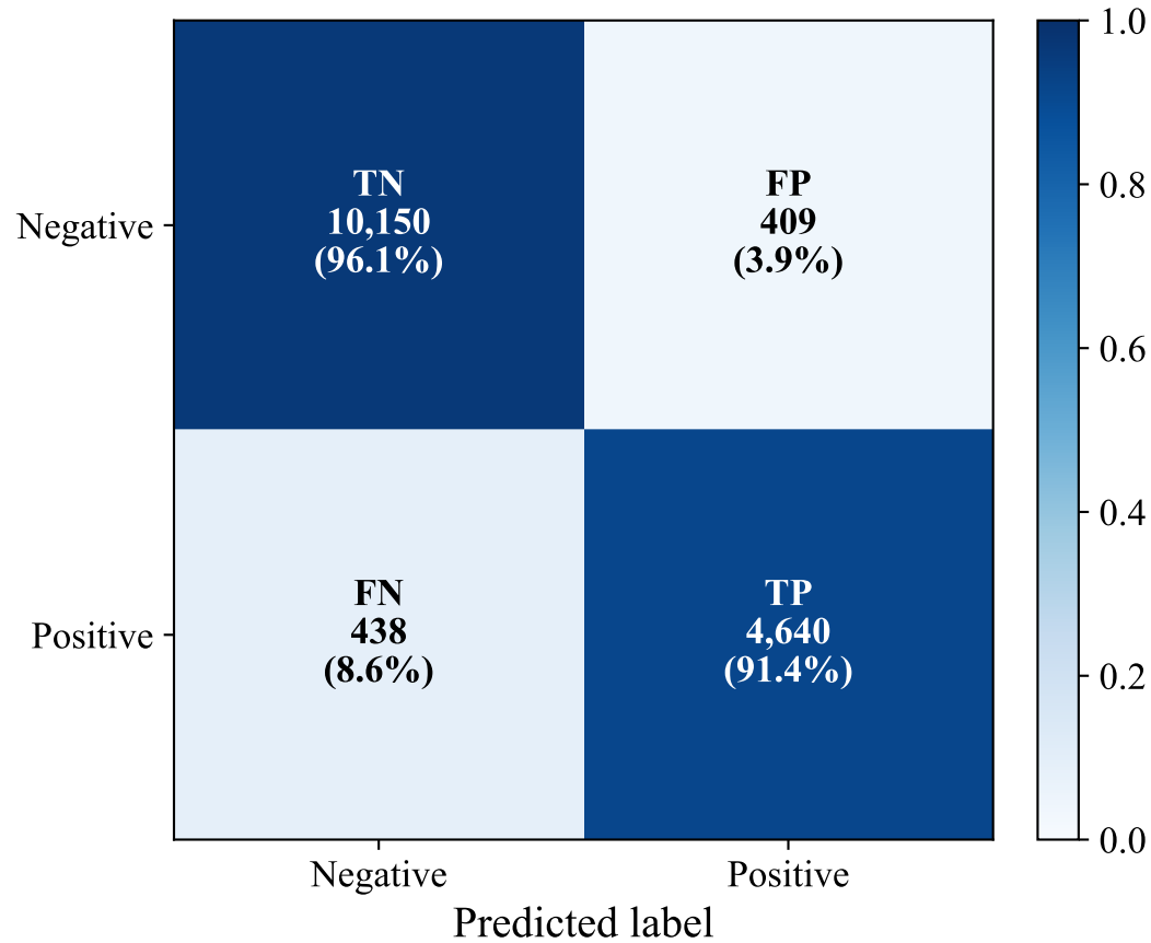
BNS
