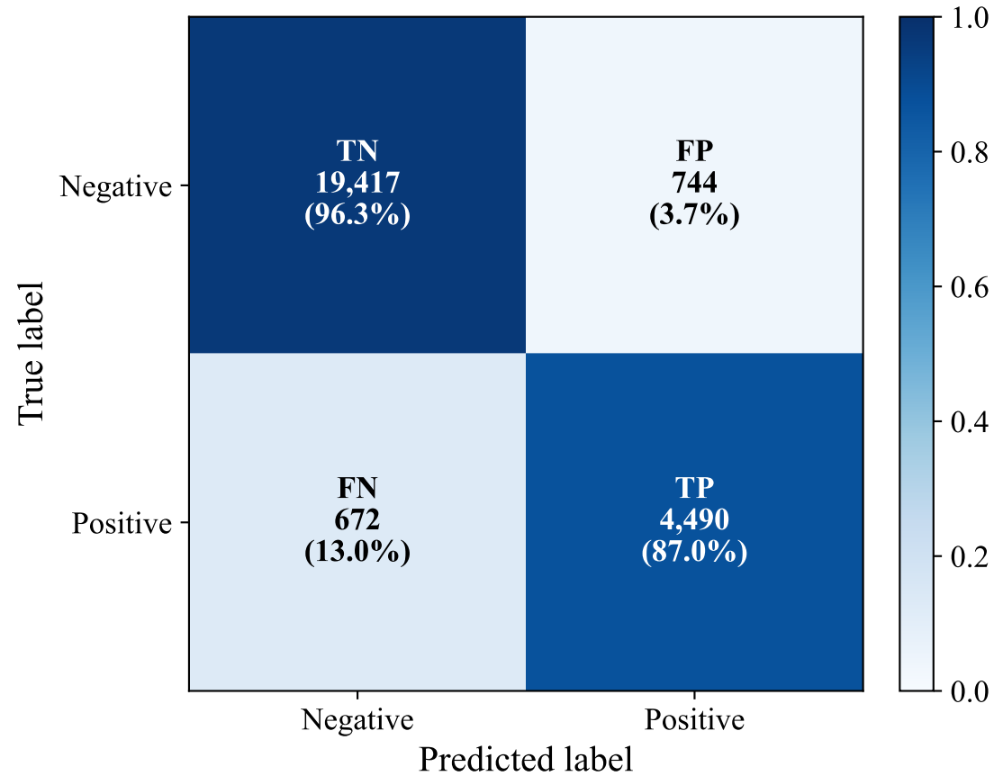
NSBH
