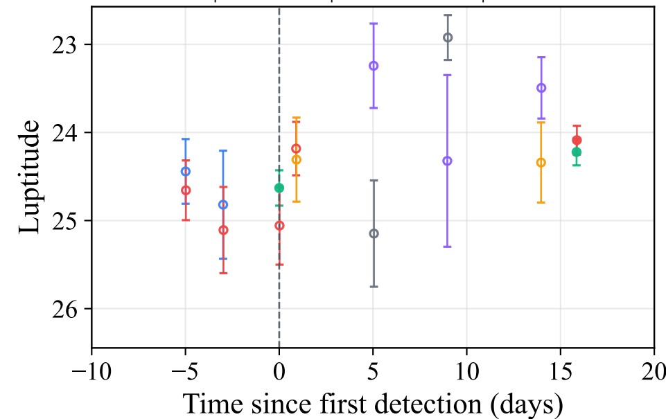
AGN | Ndet=3 | Nbands=6 | Nobs=16
