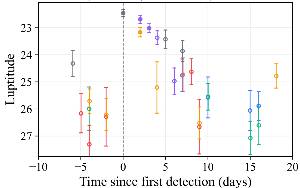
KN | Ndet=4 | Nbands=6 | Nobs=28
