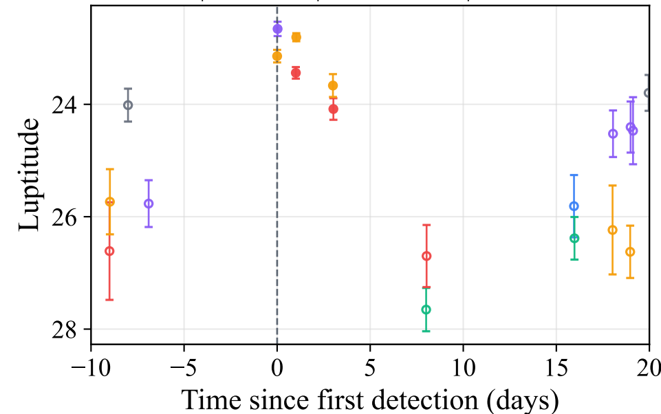
KN | Ndet=6 | Nbands=6 | Nobs=20
