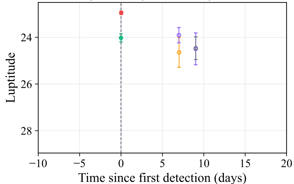
KN | Ndet=2 | Nbands=5 | Nobs=6
