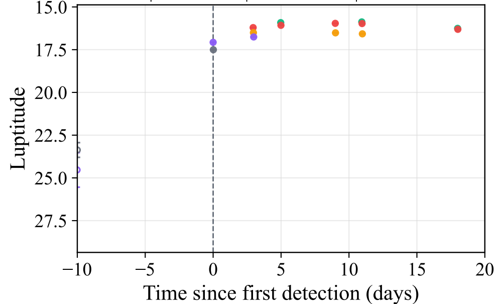
SN | Ndet=14 | Nbands=5 | Nobs=14
