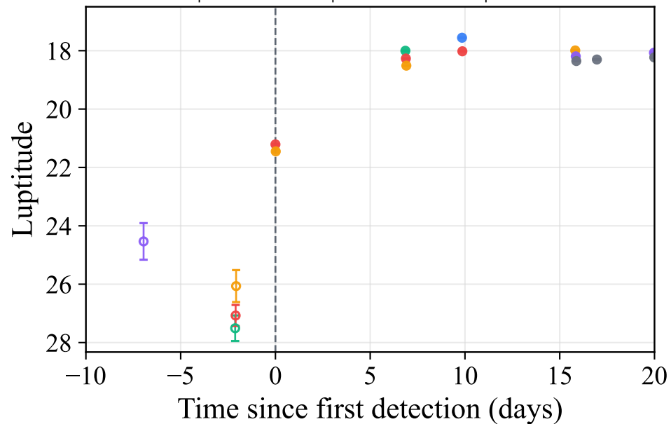
TDE | Ndet=13 | Nbands=6 | Nobs=17
