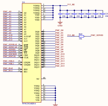
W9825G6KH-6
