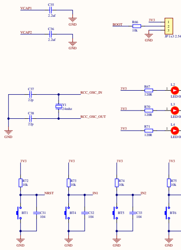
CN_STM32
