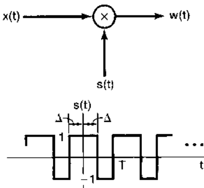
图 P7.24
