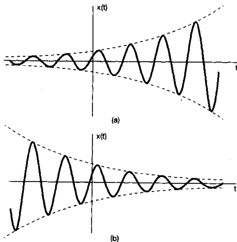
图 1.23 (a) 幅度增长的正弦信号 x(t) = Ce^{rt} \cos(\omega_0 t + \theta) , r>0 ;
