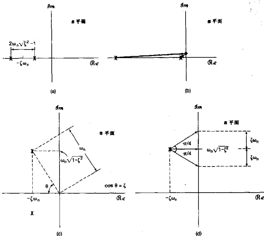
图 9.19 (a) \zeta > 1 时二阶系统的零极点图; (b) \zeta \gg 1 时的极点向量;
