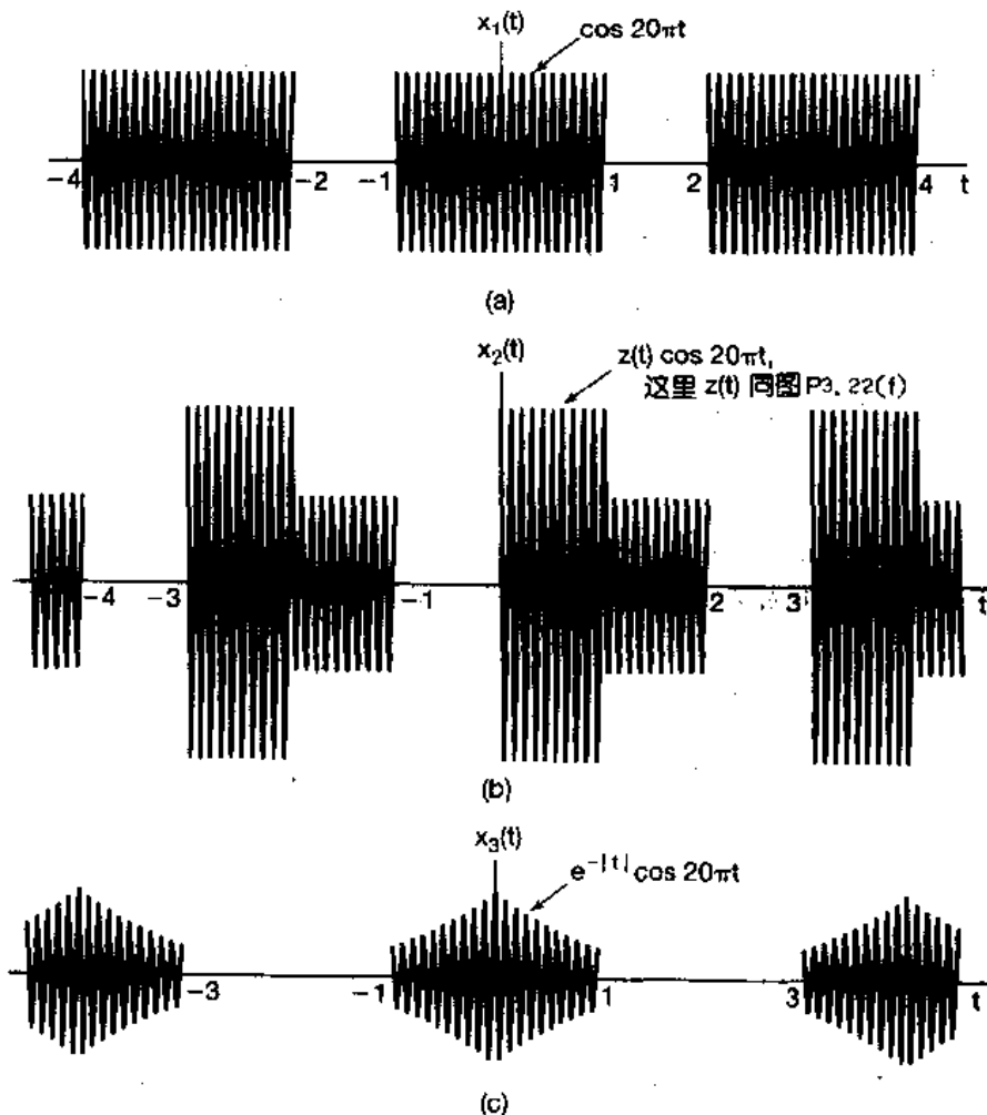
图 P3.46
