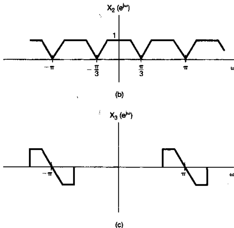
图 P5.26
