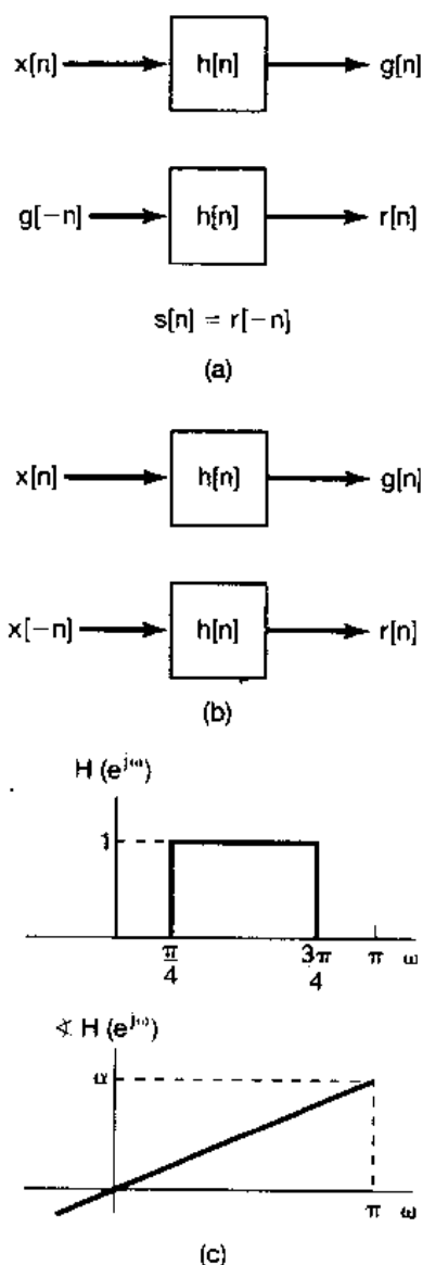
图 P6.58
