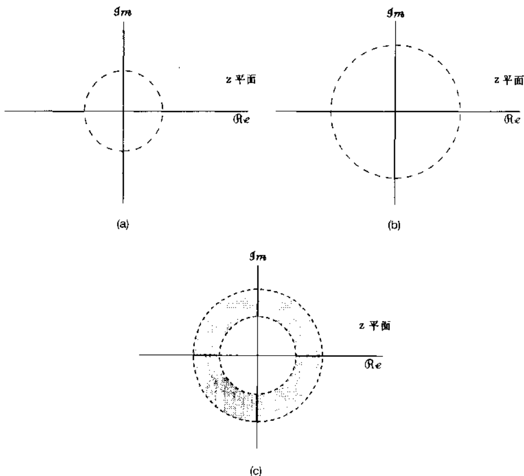
图 10.8 (a) 右边序列的 ROC; (b) 左边序列的 ROC;
