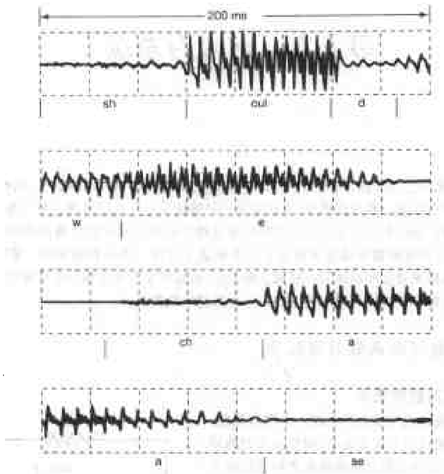
图 1.3 一个语音信号的波形[摘自“Applications of Digital Signal Processing”, A. V. Oppenheim, ed. (Englewood Cliffs, N. J. : Prentice - Hall, Inc., 1978), p. 121.]该信号代表“Should we chase”这句话的声压随时间的变化波形。图的上部相应于字“Should”, 第二行是字“we”, 最下面两行是“chase”。(图中还大致标出了每个字中逐个音的起始和结束部位)
