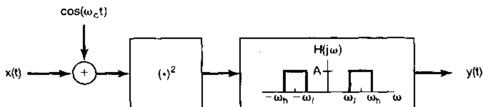
图 P8.34
