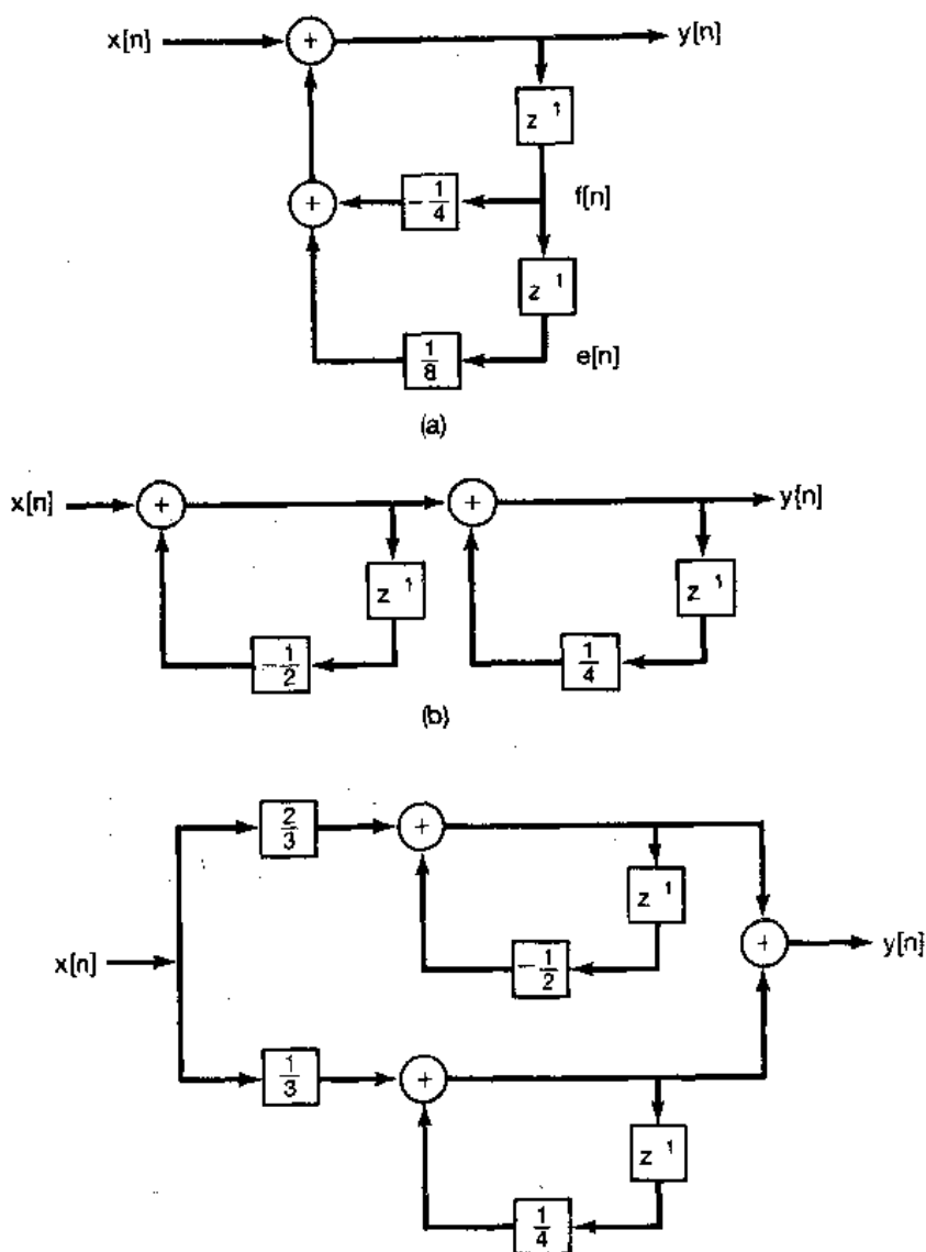
图 10.20 例 10.30 的系统方框图表示:
