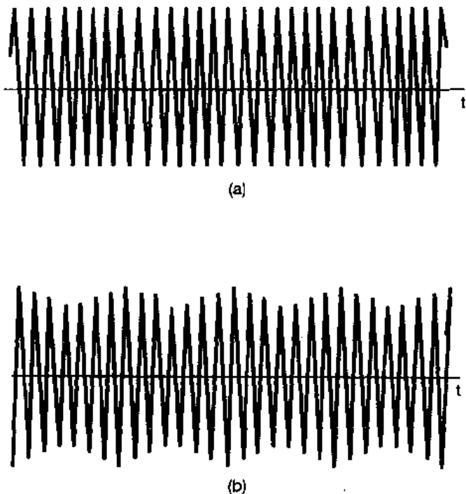
图 8.34 窄带 FM 与 AM-DSB/WC 比较:
