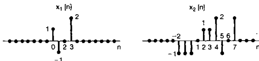
图 P5.53
