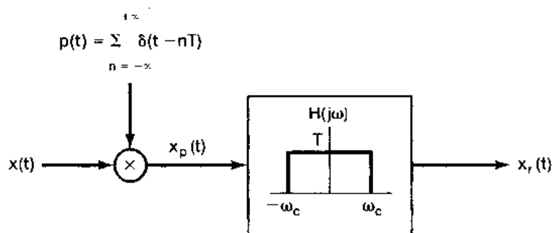
图 P7.25
