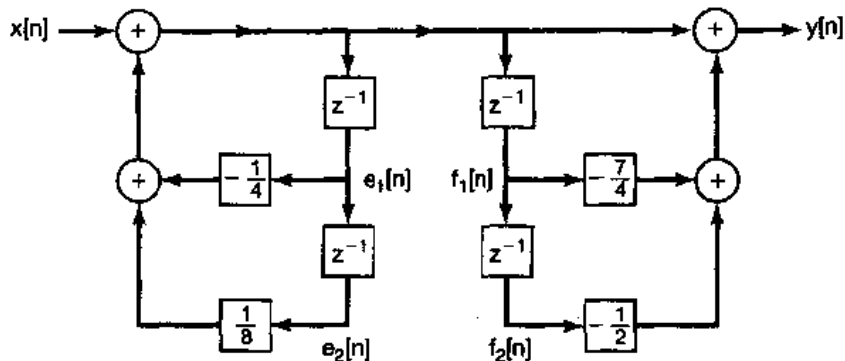
图 P10.38
