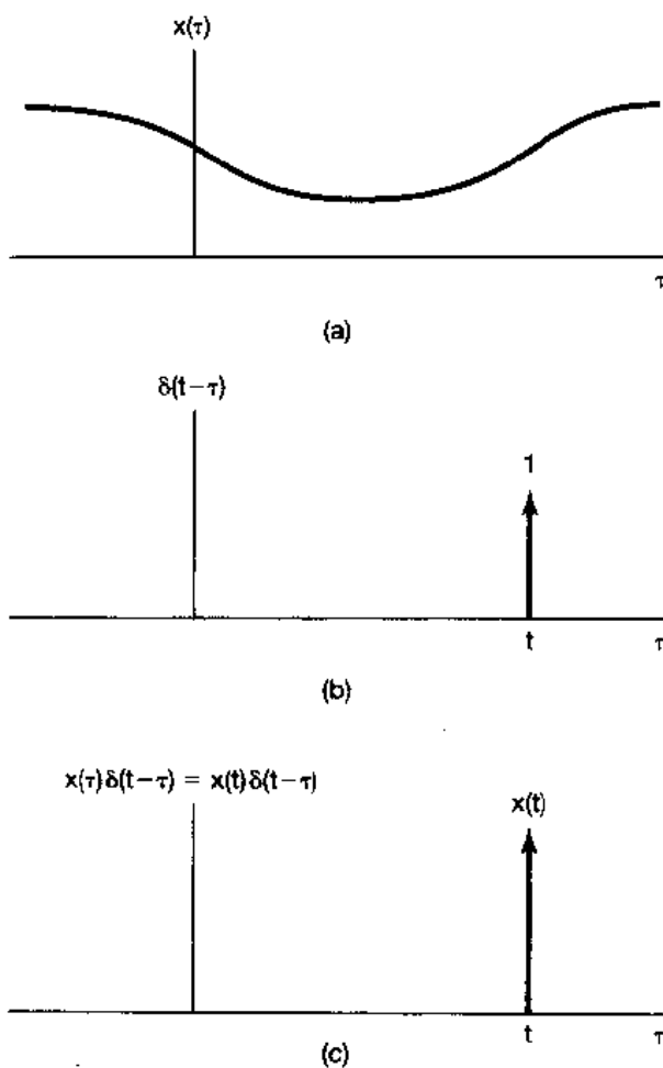
图 2.14 (a)任意信号 x(\tau) ; (b) t 固定, 作为 \tau 的函数的冲激 \delta(t - \tau) ; (c) 该二信号的乘积
