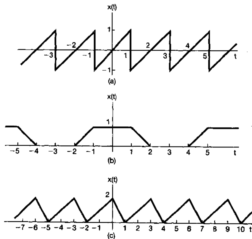
图 P3.22
