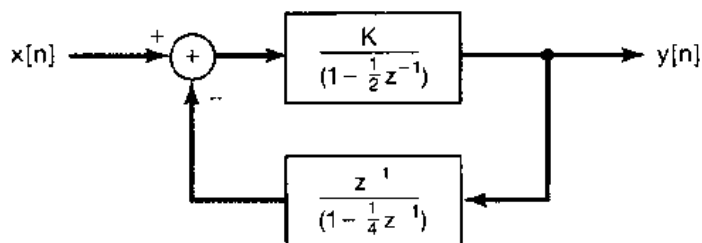
图 11.15 例 11.3 的离散时间反馈系统
