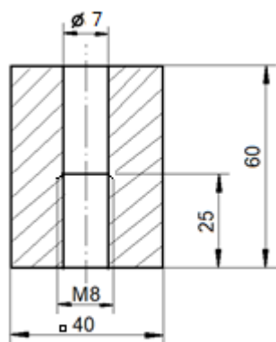
PRESJEK A - A
