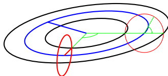
Le rayon du cercle bleu est a et le rayon du cercle rouge est b . L'angle dans le cercle rouge est u et l'angle dans le cercle bleu est v .
