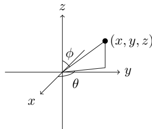
FIGURE 2.2 – Coordonnées sphériques
