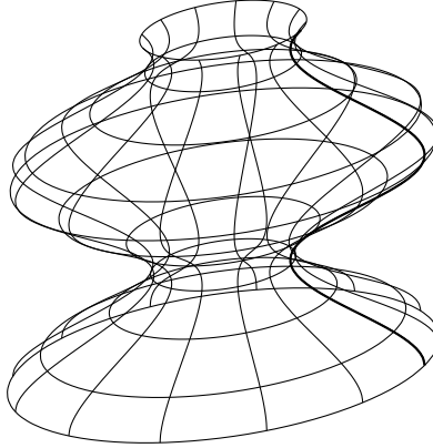
FIGURE 2.4 – Exemple de surface de révolution
