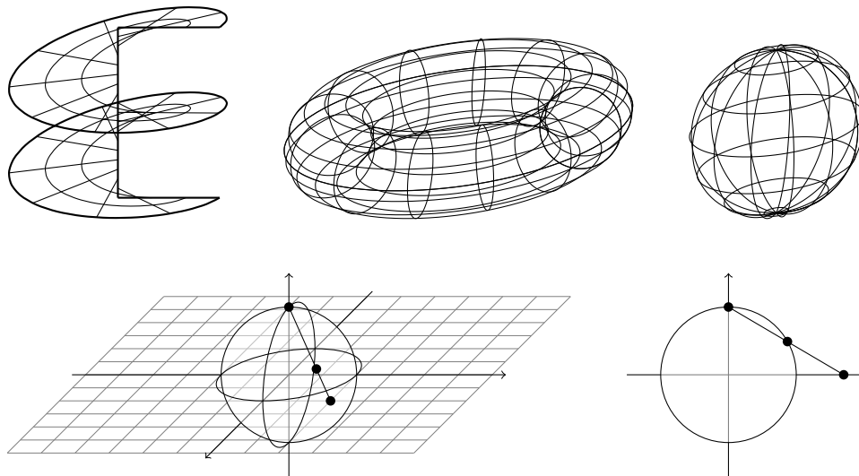
FIGURE 2.3 – Hélicoïde, tore, sphère et visualisation de la projection stéréographique
