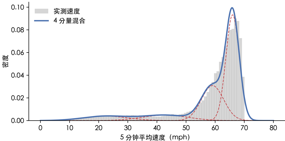
METR-LA 全部检测器速度分布的高斯混合拟合
