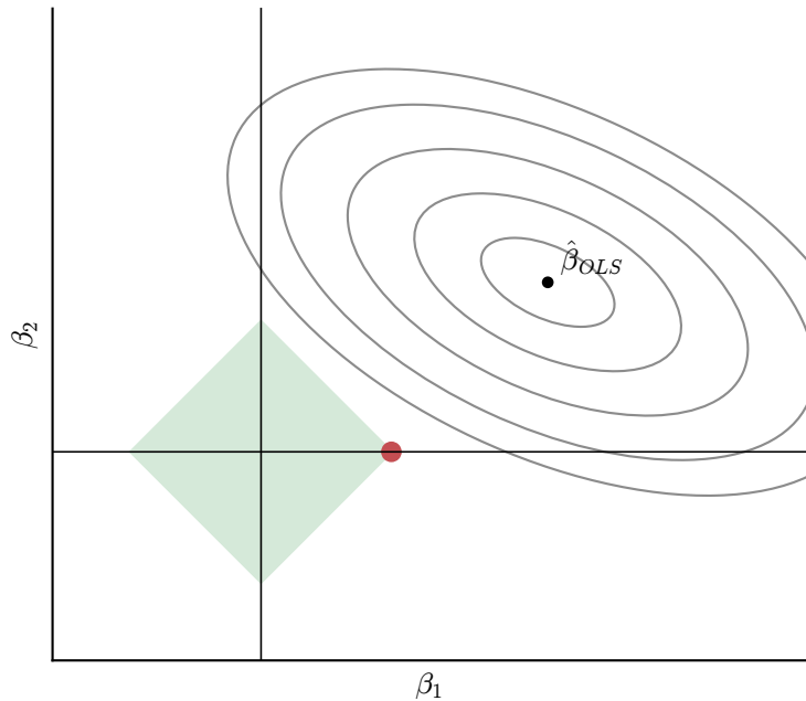
Lasso : L_1 约束 (菱形)
