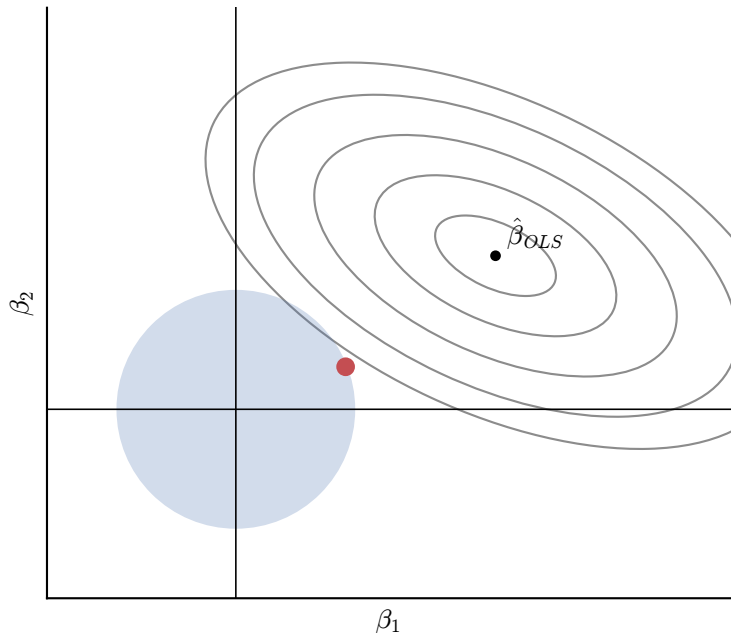
Ridge : L_2 约束 (圆)
