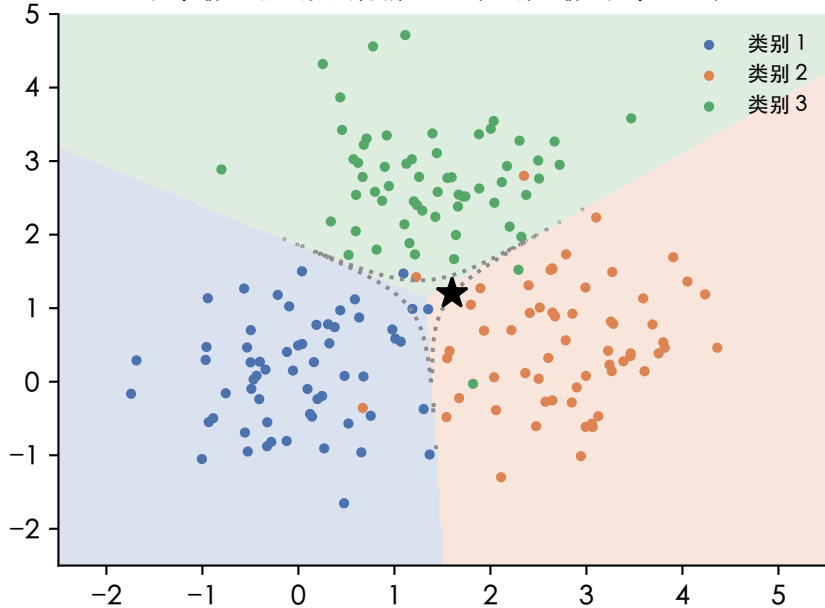
概率最大的类别形成决策区域（虚线：最大概率 = 0.5）
