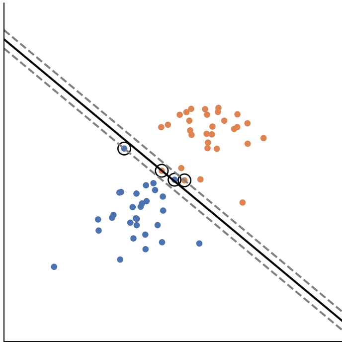
C=100 ：间隔较窄，尽量少犯错
