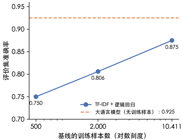
(a) 与低成本基线比较
