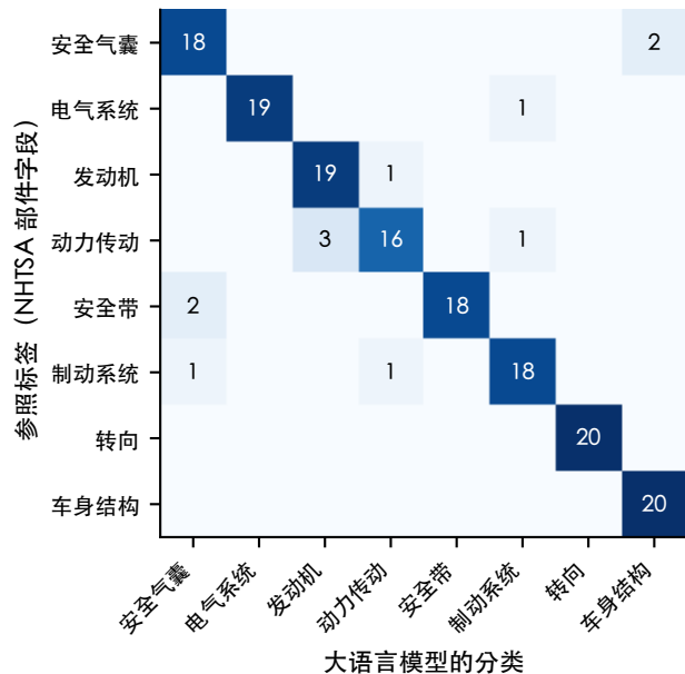
(b) 大语言模型的混淆矩阵（160 条）
