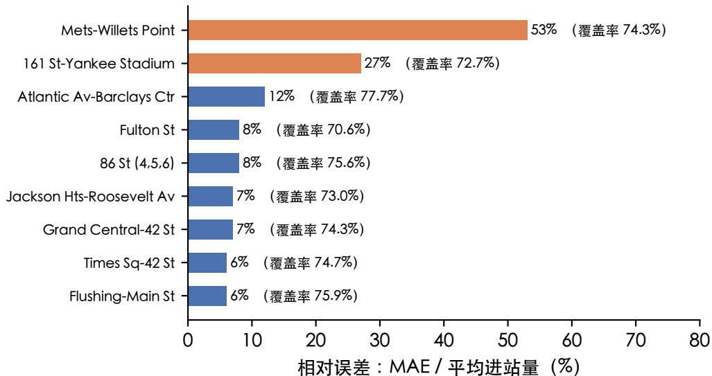
(b) 各车站的相对误差 (橙色为球场车站)
