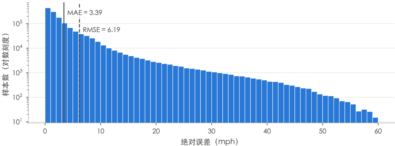
持续性基准在测试集上的绝对误差分布：2.1% 的样本误差超过 20 mph
