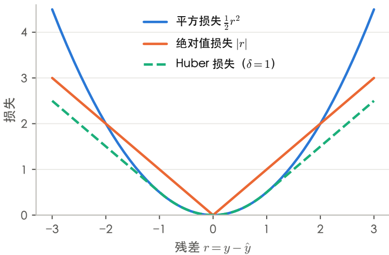
(a) 回归：大残差受到的惩罚不同
