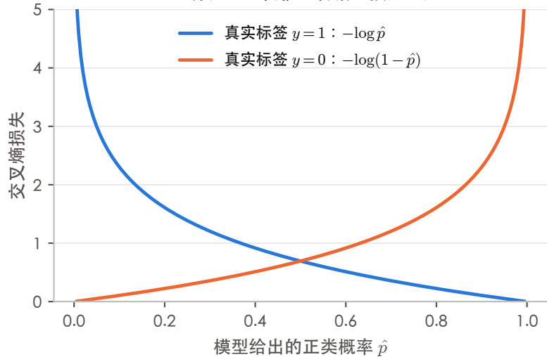
(b) 分类：越自信地答错，损失越大
