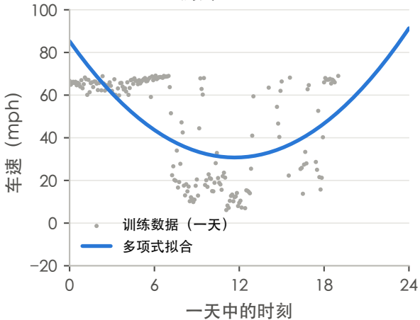
2次：训练 MAE 15.6 测试 MAE 19.5
