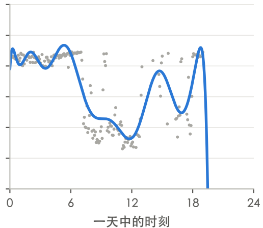
14次：训练 MAE 7.9 测试 MAE 约 2.8 万
