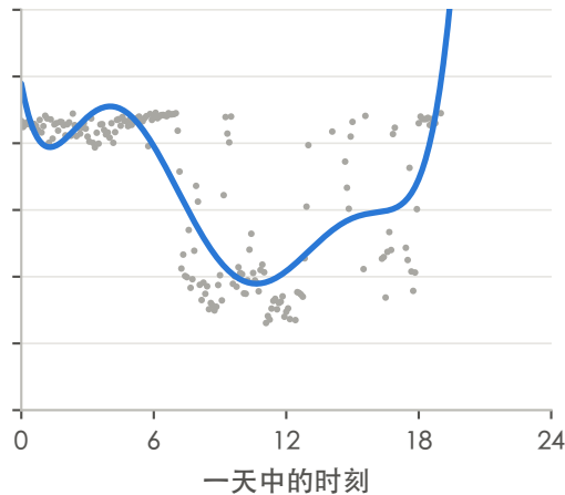
6次：训练 MAE 10.2 测试 MAE 132.3
