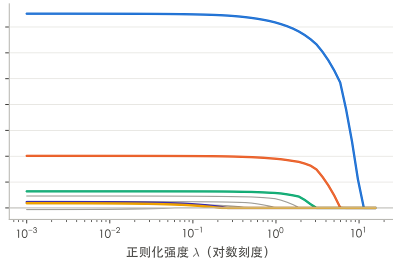
(b) Lasso：系数逐个变为零
