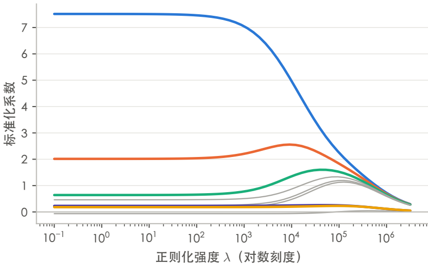
(a) 岭回归：系数整体收缩，但不为零
