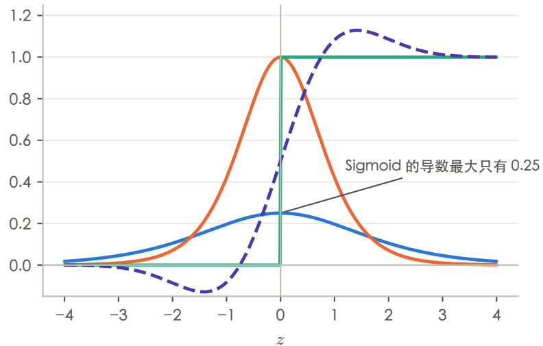
(b) 导数 g'(z) ：反向传播时梯度乘上的因子
