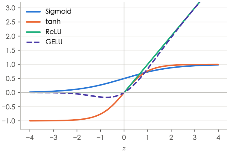
(a) 激活函数 g(z)
