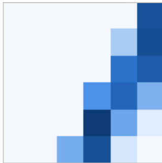
ReLU 之后
