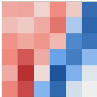
卷积结果 6×6
