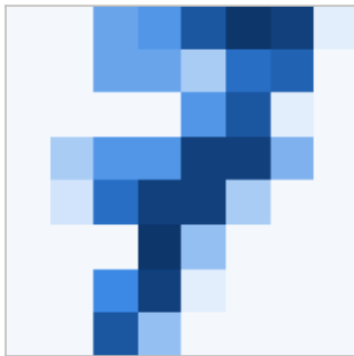
输入图像 8×8
