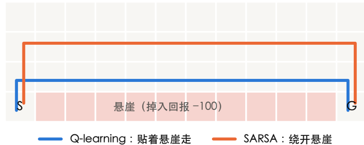
(b) 训练后的贪心路径 (种子 0)
