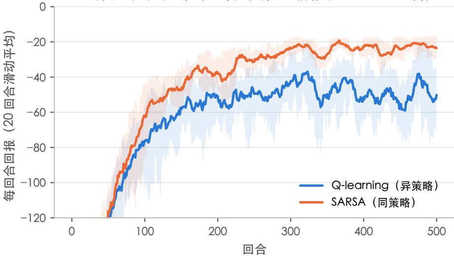
(a) 训练过程中的回报 (10 个随机种子, 阴影为 10%—90% 区间)
