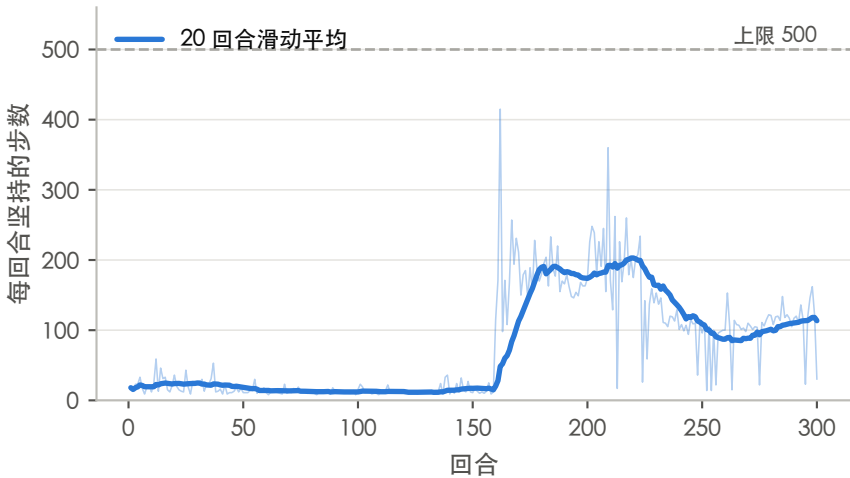
DQN (CartPole, 种子 0)
