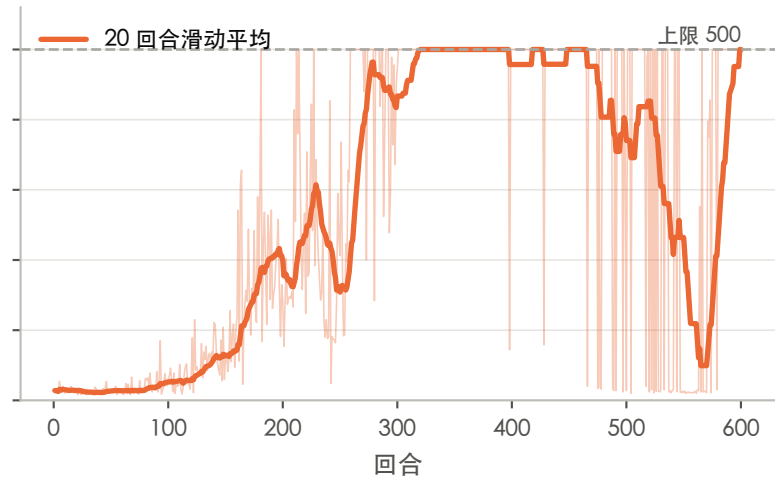
REINFORCE (CartPole, 种子 0)
