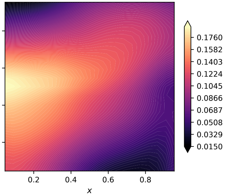
Absolute error
