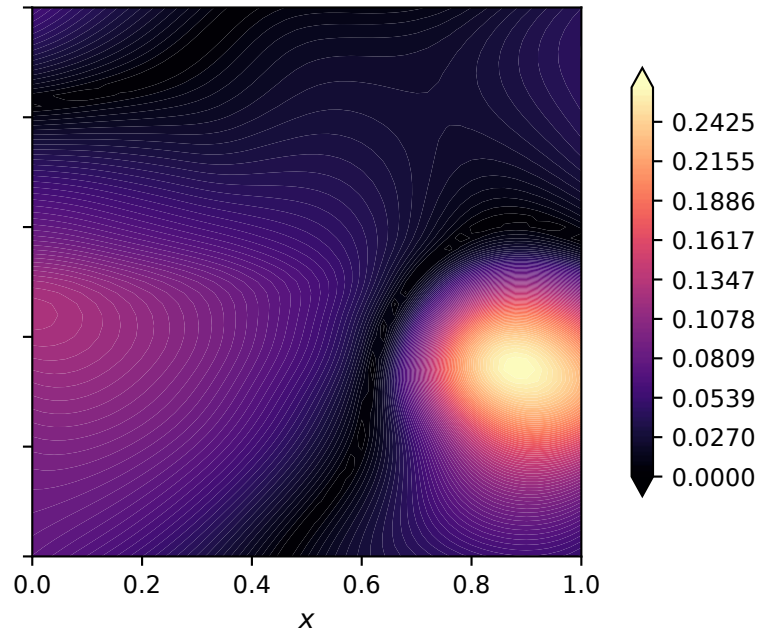
Absolute error
