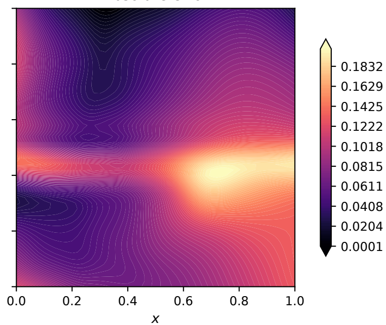
Absolute error
