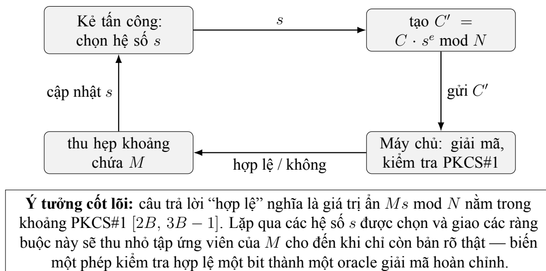
Figure 6: Tấn công Bleichenbacher là một vòng lặp phản hồi thích nghi: mỗi bit oracle thu hẹp khoảng phải chứa bản rõ.
