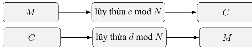
Figure 3: RSA áp dụng số mũ công khai theo chiều thuận và số mũ bí mật theo chiều nghịch.
