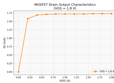
(b) V_{GS} = 1.8\text{ V}
