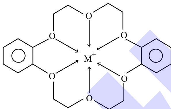
Dibenzo-18-Crown-6
