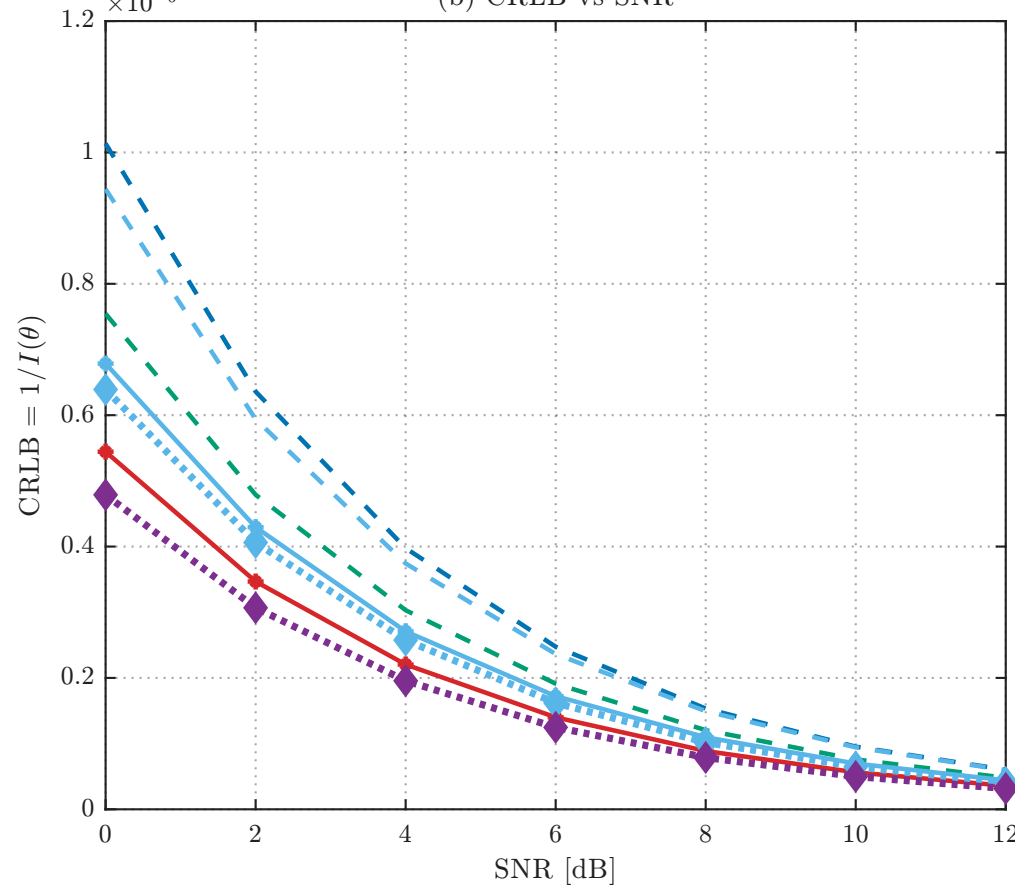
(b) CRLB vs SNR
