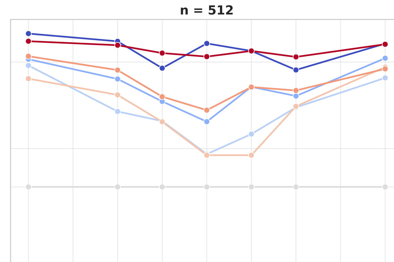
fp8_e5m2_mul_max_relative_error
