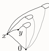
Rysunek 12: Proces uzyskiwania diagramu z grafu pokryć.
