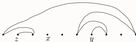
Rysunek 13: Reprezentacja lewej aktywnej pary (x, y) na linii.
