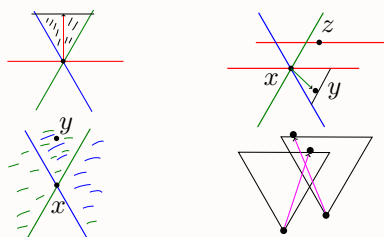
Rysunek 22: Po lewej klin z trójkątem i obszar, w którym jest krawędź. Po prawej z odgradzone od trójkąta poziomą linią i tnące się krawędzie.
