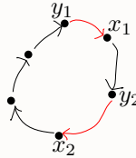
Rysunek 4: Cykl w domknięciu przechodnim.
