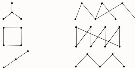
Rysunek 14: Poset incydencji cyklu to korona, a drzewa z dwoma dziećmi – pajak.
