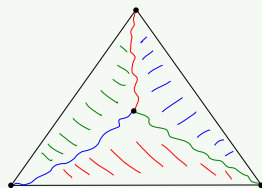
Rysunek 20: Podział grafu na trzy regiony.
