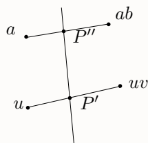
Rysunek 15: Przecięcie odcinków z prostą równoległą do (1, 1, 1) przechodzącą przez P .
