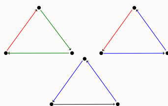
Rysunek 19: Kolorowania C dające sprzeczność.
