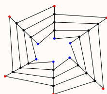
Rysunek 8: Koło Trottera z 1978.
