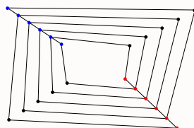
Rysunek 6: Przykład Kelly'ego z 1981.
