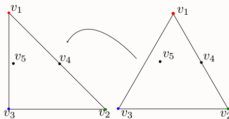
Rysunek 23: Przejście z trójkąta równobocznego w prostokątny.
