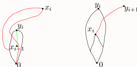
Rysunek 11: Sprzeczności wykazane dla Q_{\text{left}} i Q_{\text{under}} .
