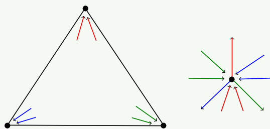
Rysunek 17: Warunki dla wierzchołków w lesie Schnydera.
