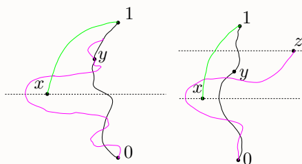
Rysunek 9: Jeśli x w przedstawionych sytuacjach musi być porównywalny z y lub z .
