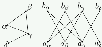
Rysunek 5: Przykład grafu i jego posetu sąsiedztwa.
