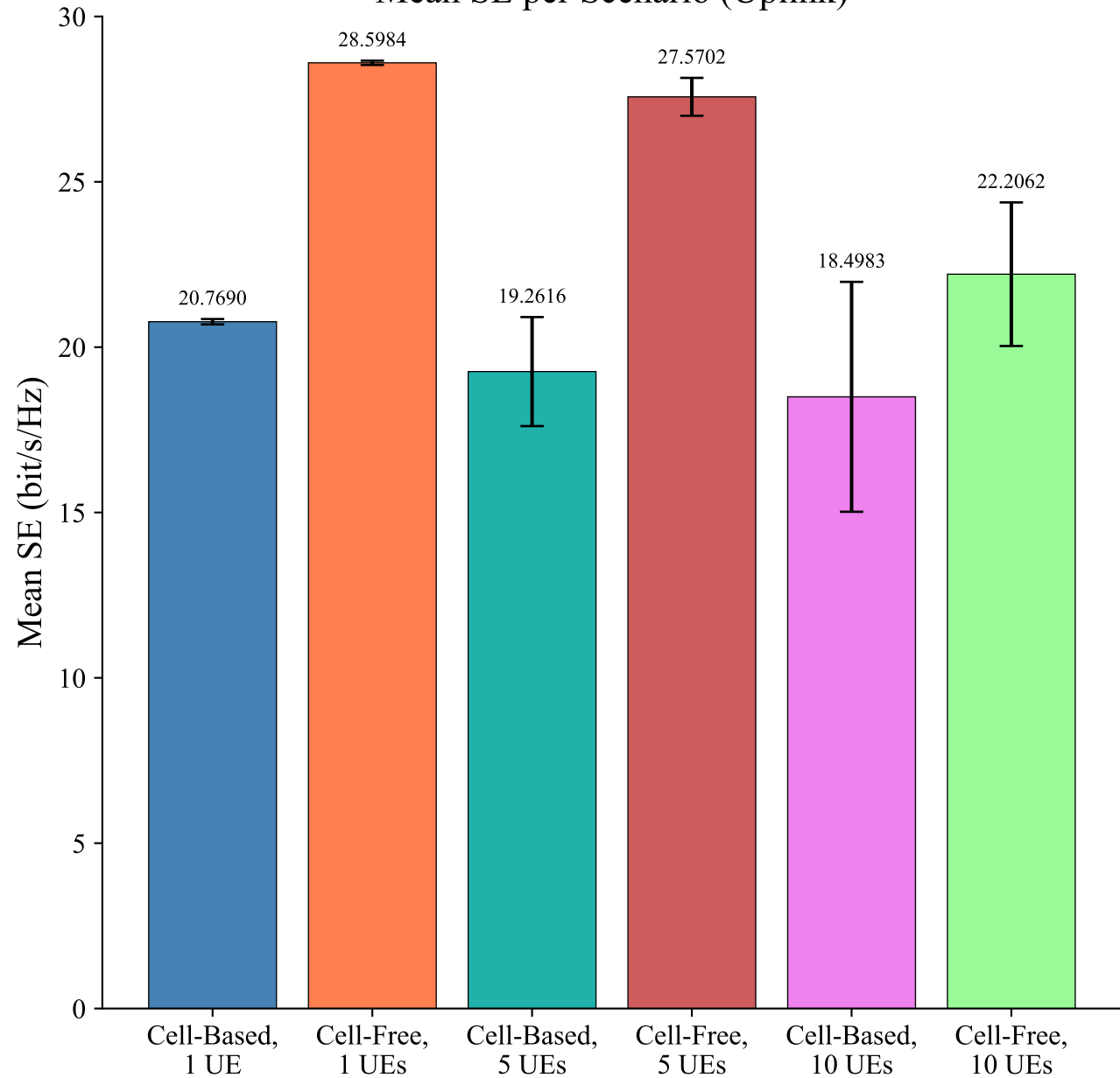
Mean SE per Scenario (Uplink)
