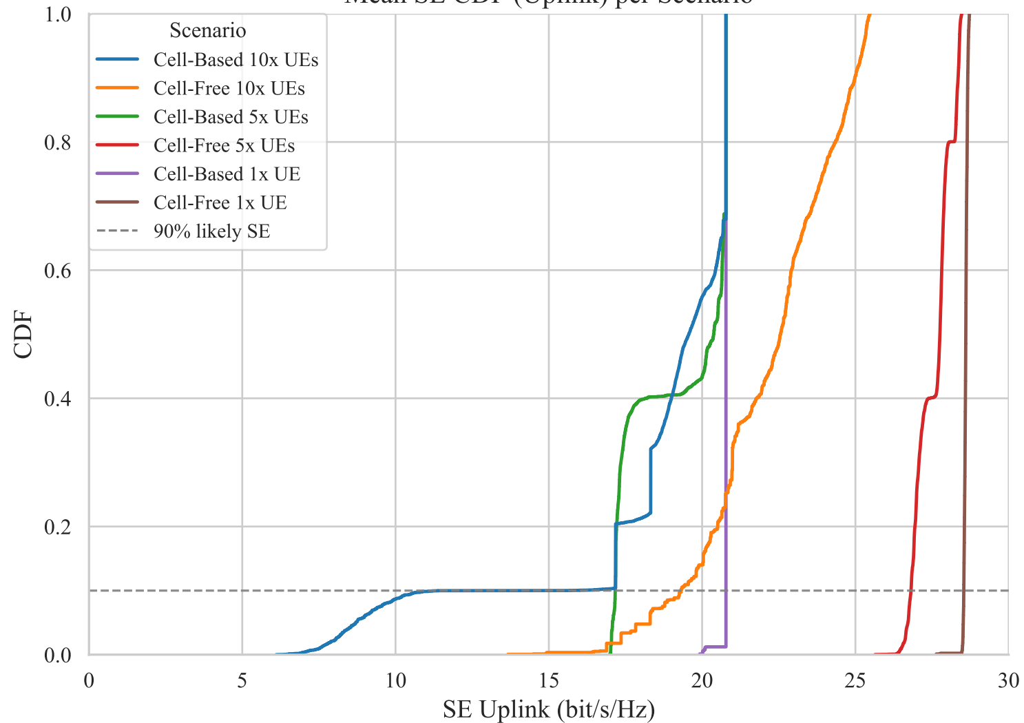
Mean SE CDF (Uplink) per Scenario
