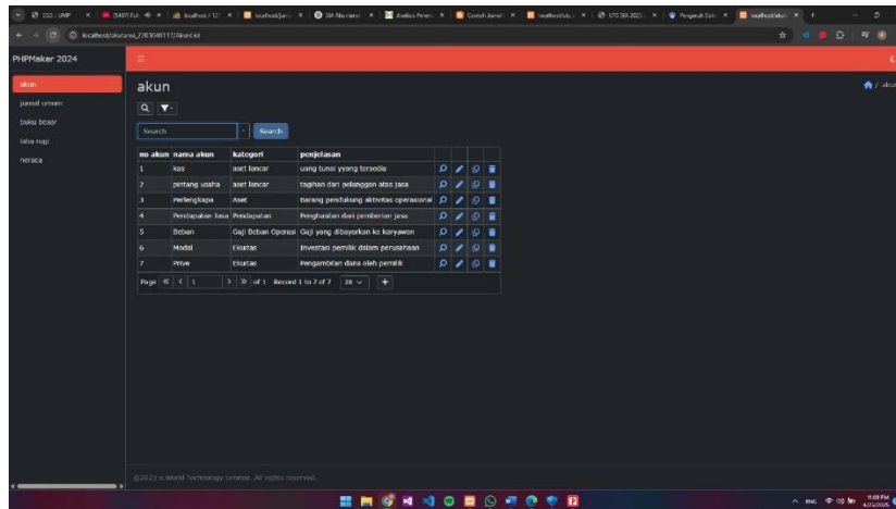
Gambar 1 Menampilkan akun
