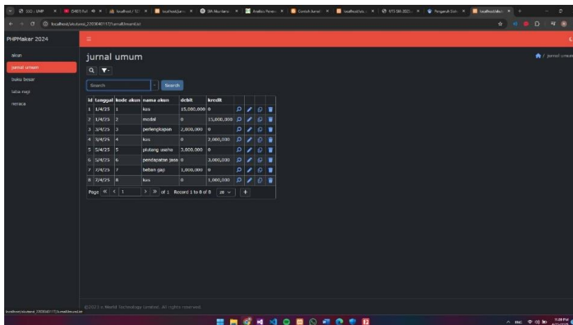
Gambar 2 Menampilkan Jurnal
